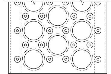
Perf-O-Grip 2
